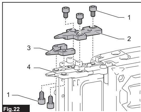
► 1. Perno hexagonal 2. Cubierta de la guía de clavado 3. Cubierta superior de contacto 4. Guía de clavado
