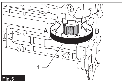
Fig.5 ► 1. Ajustador
