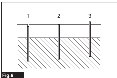
Fig.6 ► 1. Demasiado profundo 2. Profundidad correcta 3. Demasiado superficial
